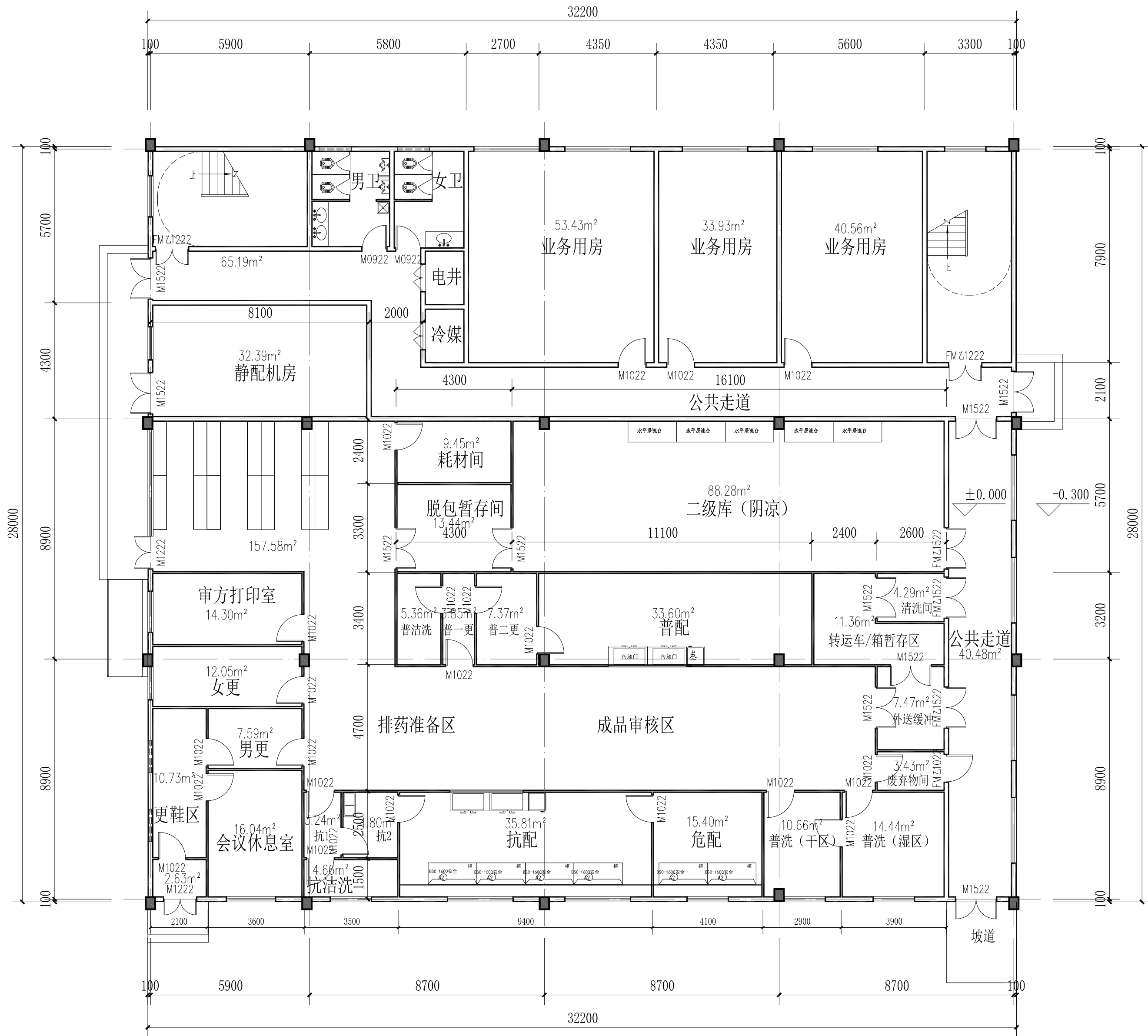
一层平面图 1:100
