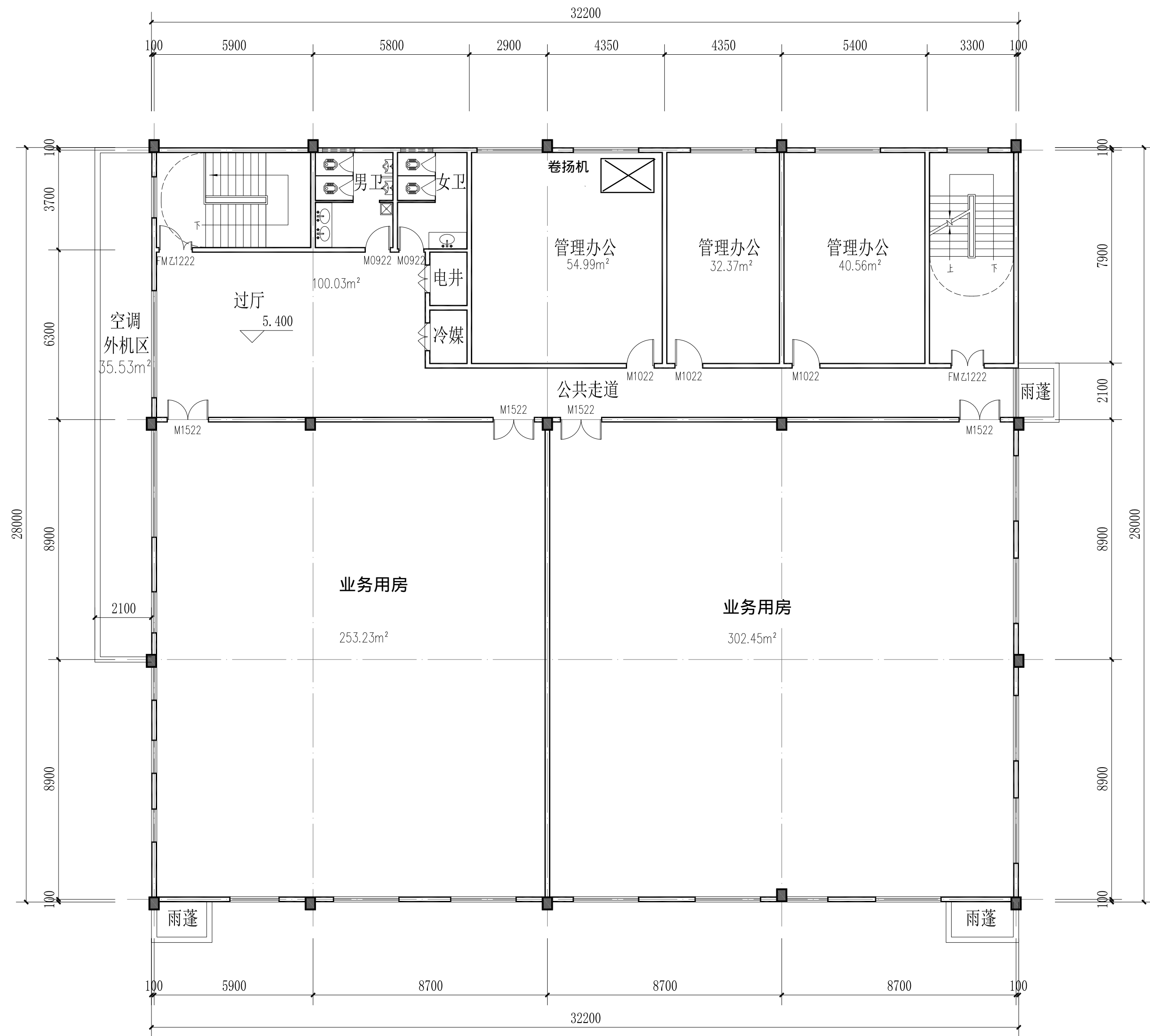
二层平面图 1:100
